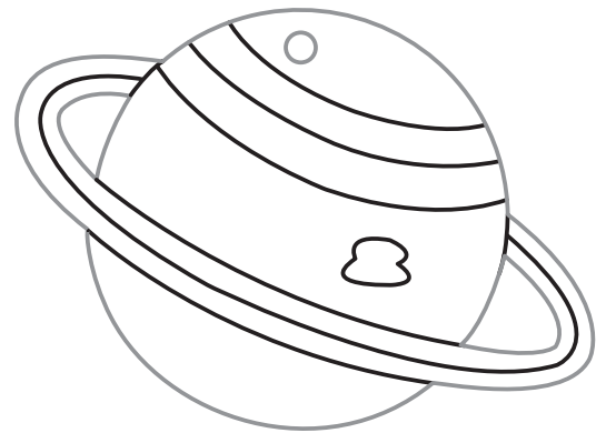
Uranus
