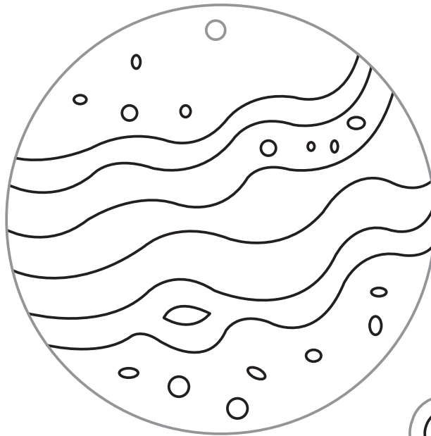
Jupiter
